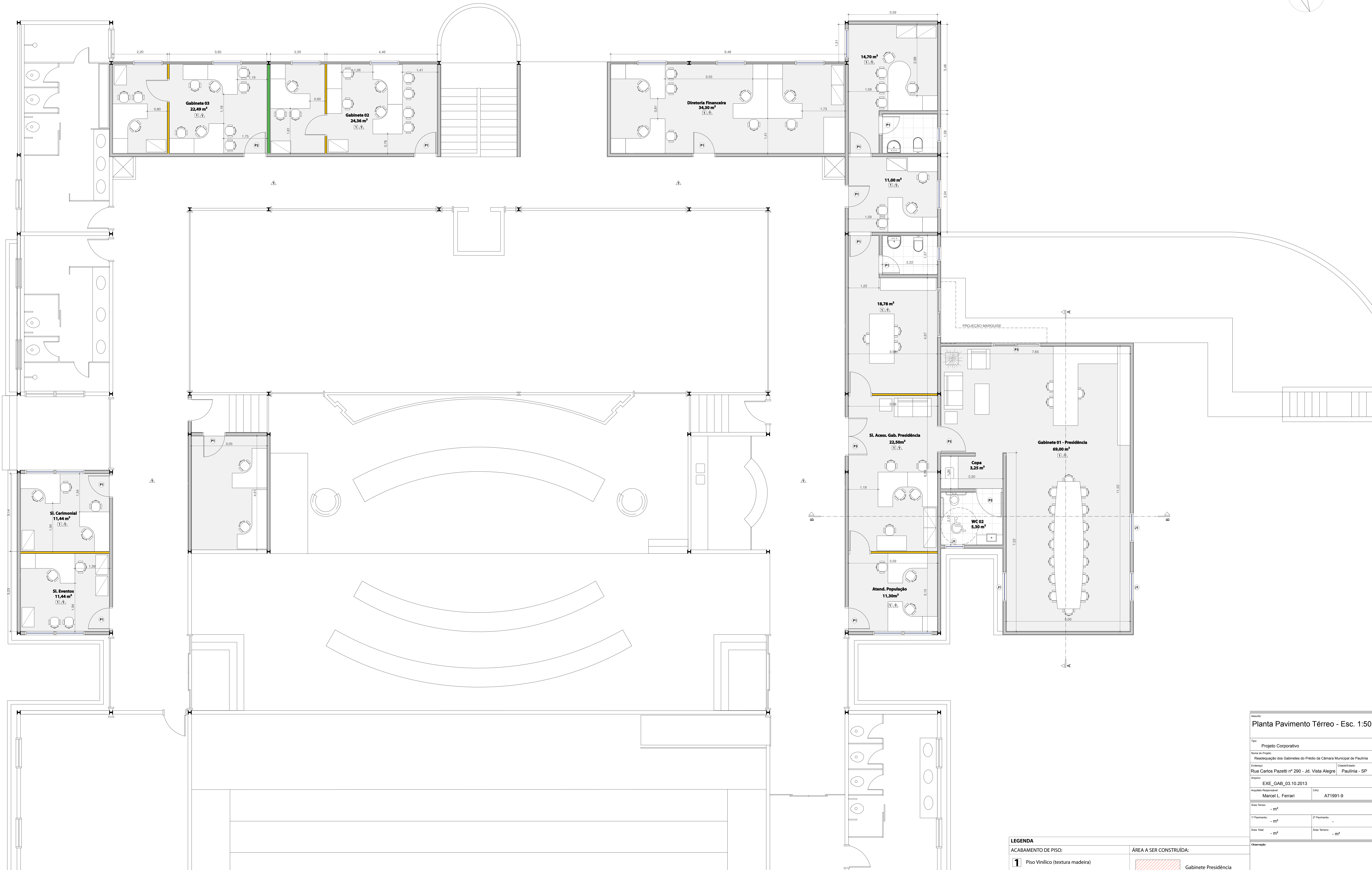
Planta Pavimento Térreo escala 1:50
